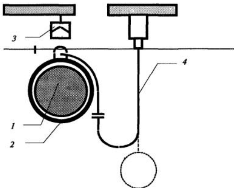
Рис. 7. Схема испытания пояса динамической нагрузкой:
