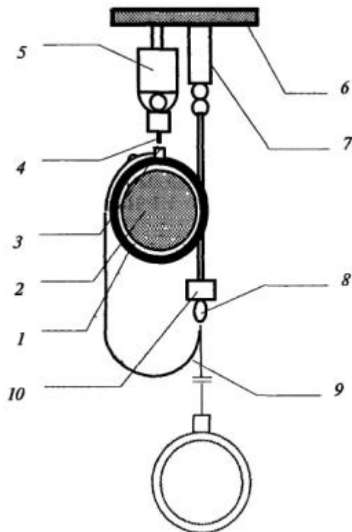
Рис. 8. Схема установки для определения усилия при динамическом рывке: 1 - пояс; 2 - груз; 3 - страховочное кольцо; 4 - разъёмная серьга; 5 – расцепляющее устройство; 6 - жесткая опора; 7 - штанга; 8 - карабин пожарный; 9 - фал; 10 - датчик
