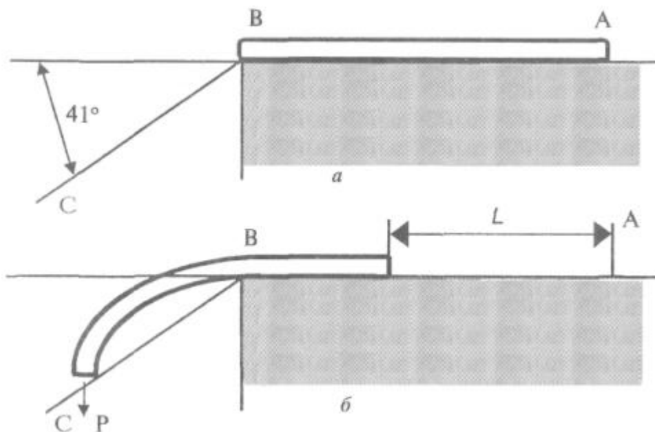
Рис. 5. Схема определения жесткости фала
